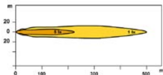
Fjärrljusbild
