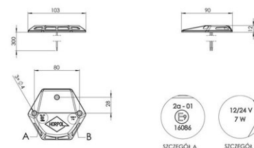
Lampa ostrzegawcza na winę, diodowa 7W 12/24V HOR 80 [LDO 2135] Warning LED light for tail lift, 7W 12/24V HOR 80 [LDO 2135]
