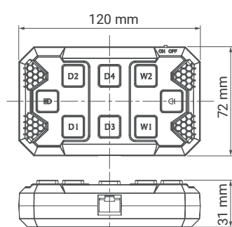
Kontrollpanel
