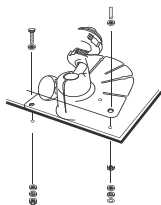
1] Bildskärmsfäste Standard
