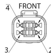
DT-Kontakt 4-pol, hane
